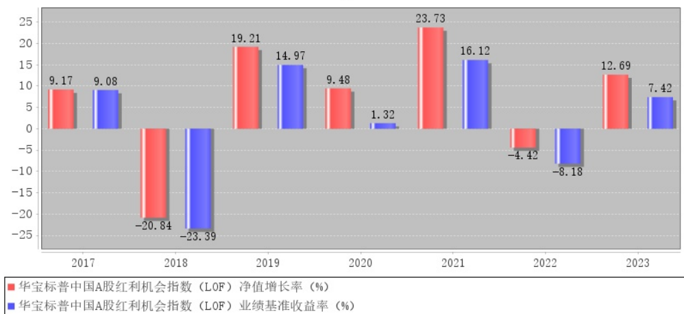
华宝标普中国A股红利机会指数 (LOF) 每年净值增长率与同期业绩比较基准收益率的对比图
